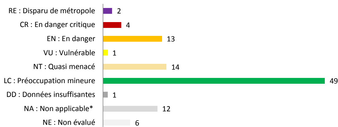
Figure 2 : Résultat de l'évaluation des 102 taxons de la liste nationale : catégories de la Liste rouge et autres catégories, et nombre de taxons par catégorie. *Taxons introduits après 1500 ou présents de façon occasionnelle ou marginale.
