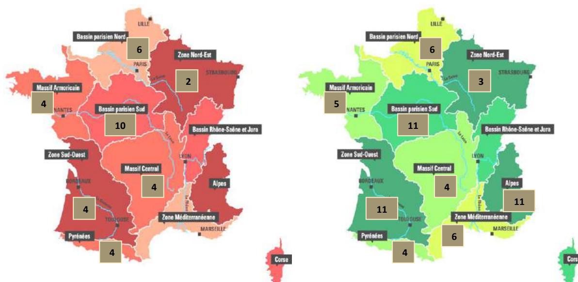
Figure 7: Nombre d'espèces de la liste nationale des plantes messicoles bénéficiant de la marque « Vraies messicoles » (à gauche) et de la marque « Végétal local » (à droite) dans chacune des régions d'origine définies par les marques.
