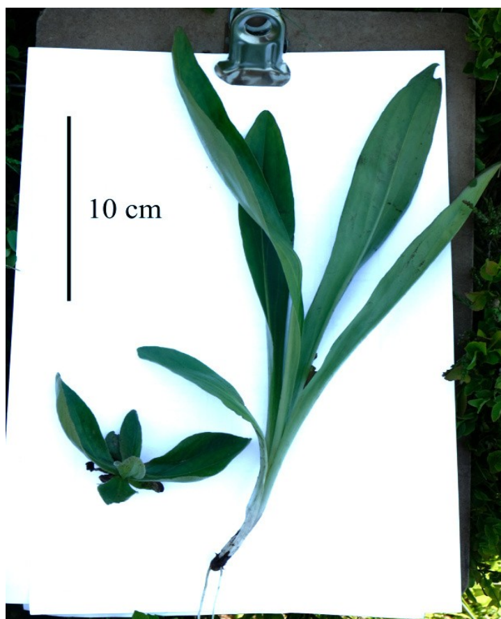
Figure 3 : Photographie de deux rosettes d'arnica prélevées dans la même population à quelques mètres de distance, mais dans un environnement végétal distinct : à gauche, sur un sol pratiquement nu, et à droite, parmi des myrtilliers hauts d'environ 30 cm de haut
