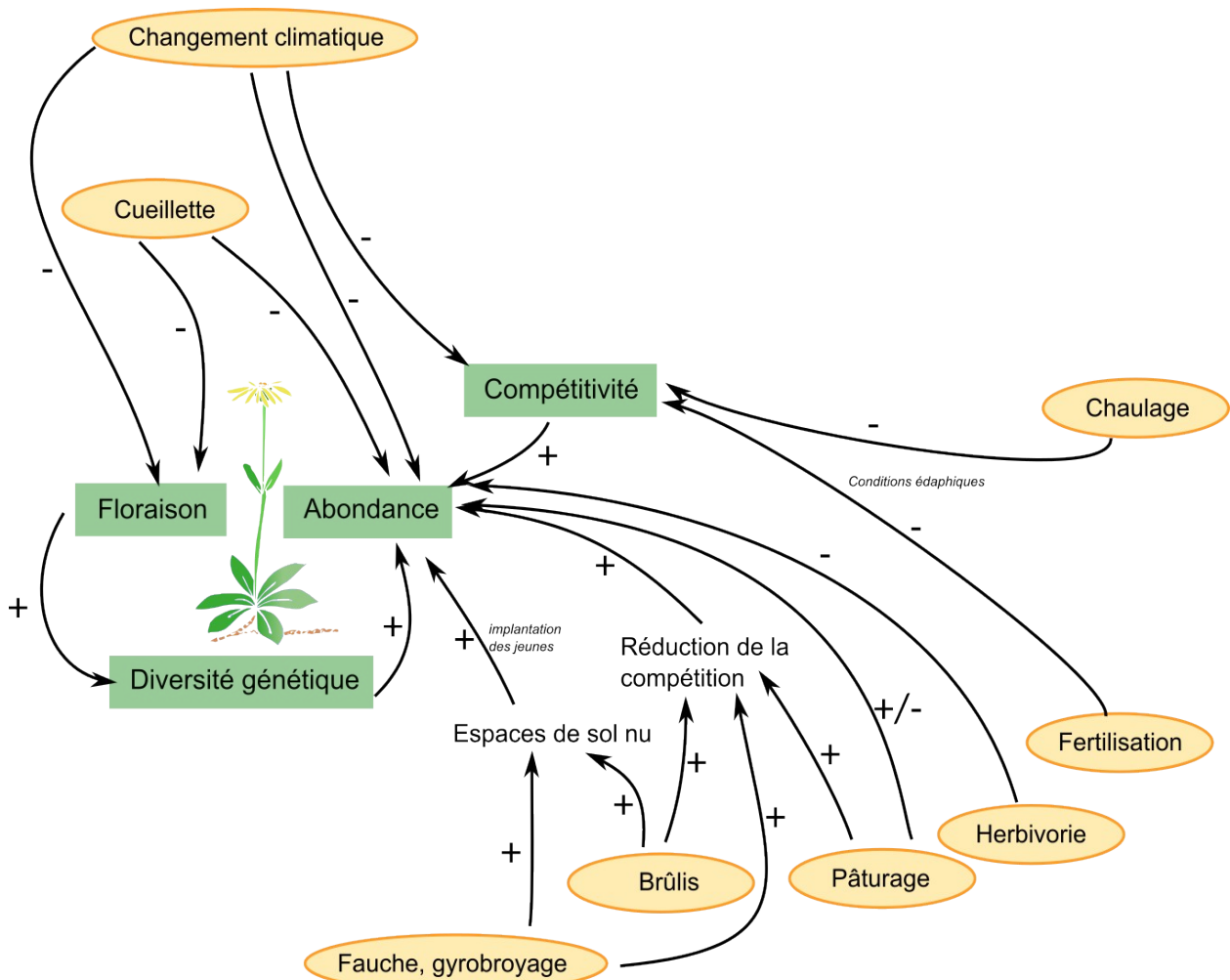
Figure 5 : Schéma des différents facteurs influant sur la présence et l'abondance de l'arnica des montagnes
