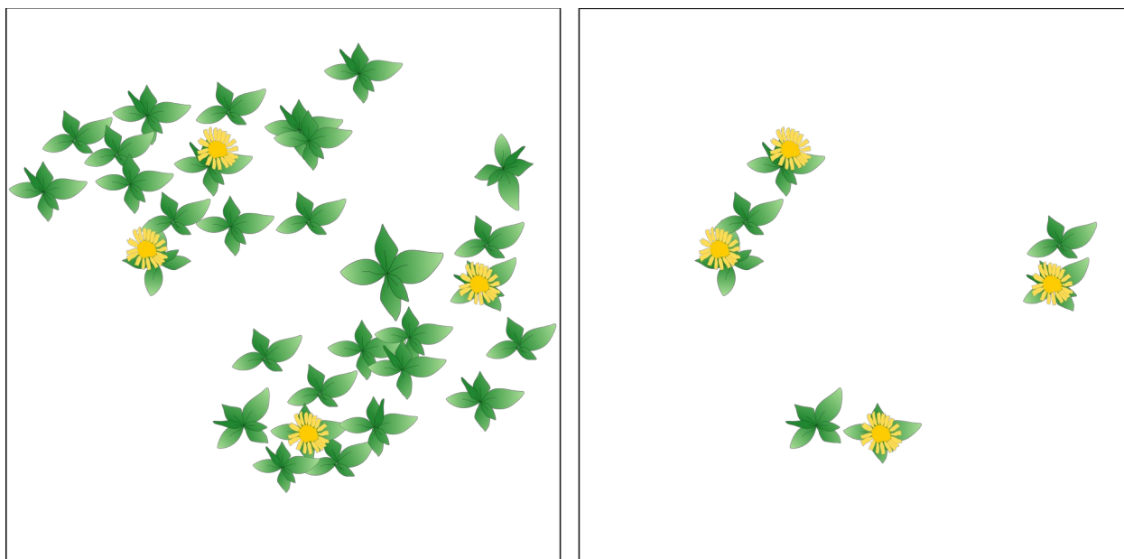
Figure 22 : Deux situations différentes où la ressource cueillable est la même (4 capitules ou rosettes fleuris) mais l'impact attendu sur la plante est distinct, puisque le nombre total de rosettes diffère. Cela illustre l'importance des suivis intégrant la densité de rosettes non fleuris.
