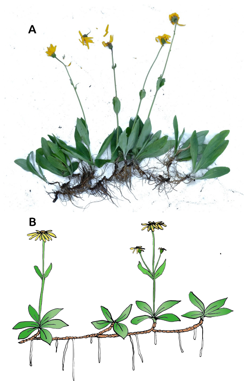
Figure 2 : En haut, photographie d'un individu d'arnica avec ses multiples rosettes connectées par le rhizome souterrain. En bas, schéma d'un individu d'arnica
