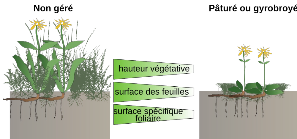
Figure 24 : Schéma de la variation des traits foliaires de l'arnica en fonction de la gestion, à partir de données collectées dans les Monts d'Ardèche. Modifié de Locqueville (2023).
