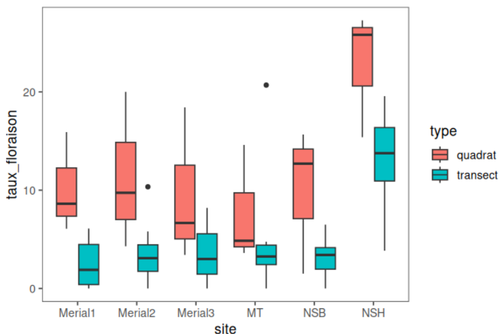
Figure 17 : Boîte à moustache du taux de floraison issus des relevés manuels du CBNPMP sur les différentes parties du site du col de Pailhères. On constate que le taux de floraison est plus élevé dans les quadrats sélectionnés que dans le transect
