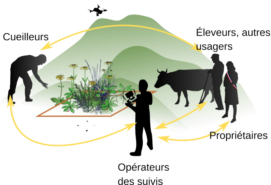
Figure 25 : Importance de la collaboration entre acteurs pour la mise en place de suivis et d'expérimentations
