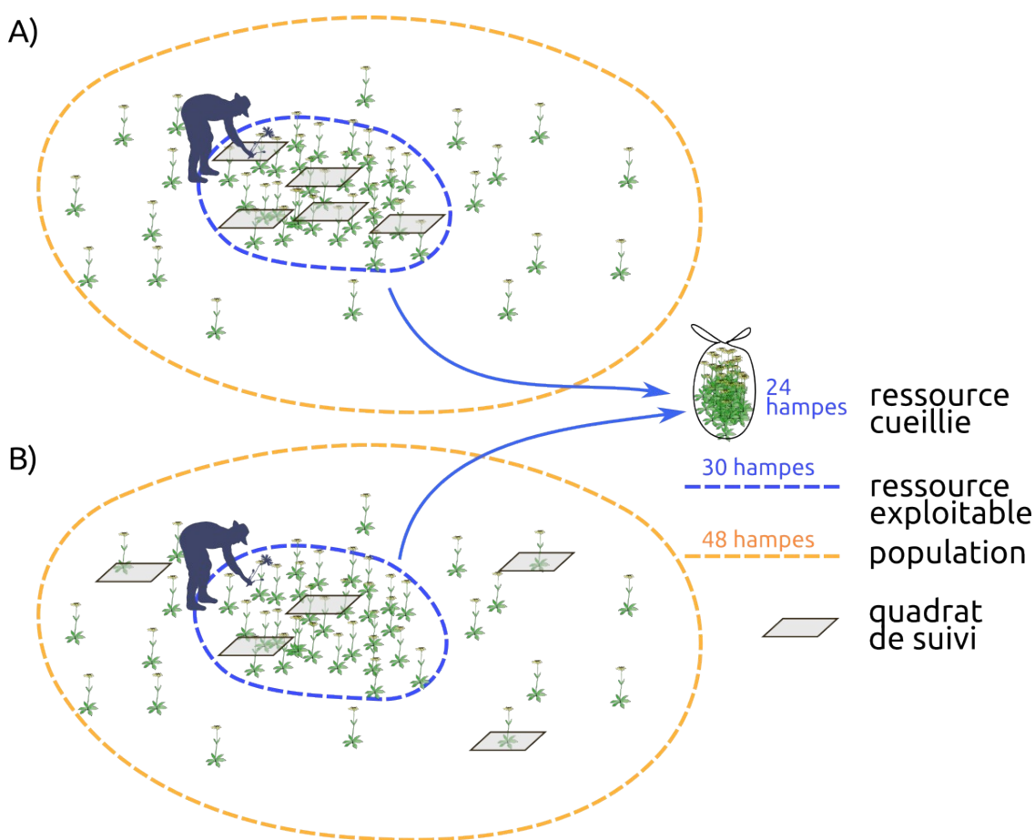
Figure 18 : Schéma de la différence entre ressource exploitable (en bleu) et population (en orange) permettant de visualiser l'effet de la spatialisation des suivis. Dans le scénario A, les suivis sont positionnés uniquement dans la zone cueillable, et conduisent à détecter une pression de cueillette de 80% (24 hampes sur 30). Dans le scénario B, les suivis sont positionnés dans l'ensemble de la population du site, conduisant à détecter une pression de cueillette de 50% (24 hampes sur 48).
