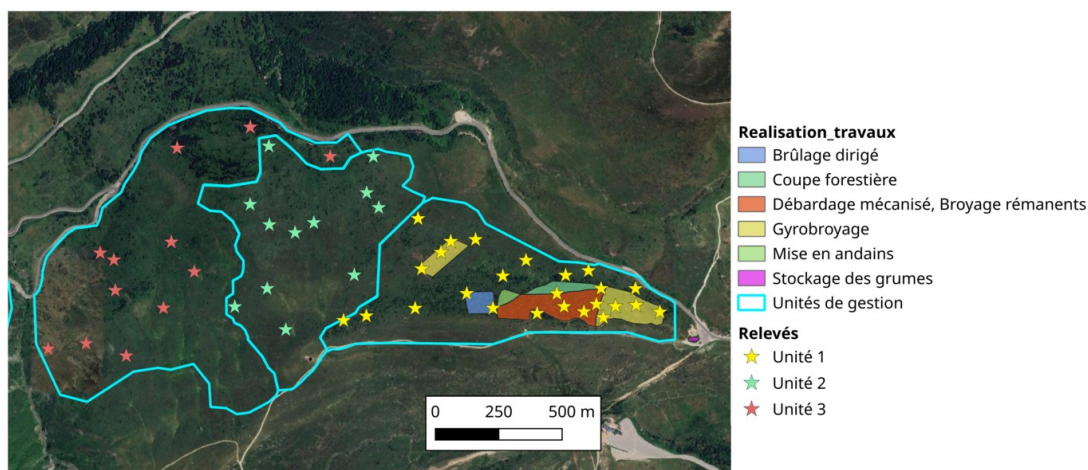
Figure 14 : Cartographie des suivis (étoiles) et des travaux effectués sur le site de cueillette de Porté-Puymorens. Les suivis des unités 1 et 2 sont réalisés annuellement, et tous les 5 ans pour les unités 3 et 4
