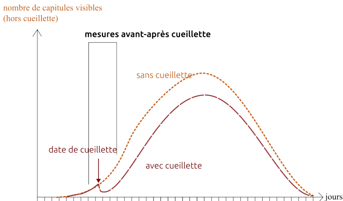
Figure 21: Graphique montrant l'influence de la date de comptage sur l'estimation de la pression de cueillette. Dans cette configuration où la cueillette a lieu bien avant l'optimum de floraison, le comptage après cueillette donne davantage de capitules qu'avant cueillette, du fait de la dynamique de la ressource.
