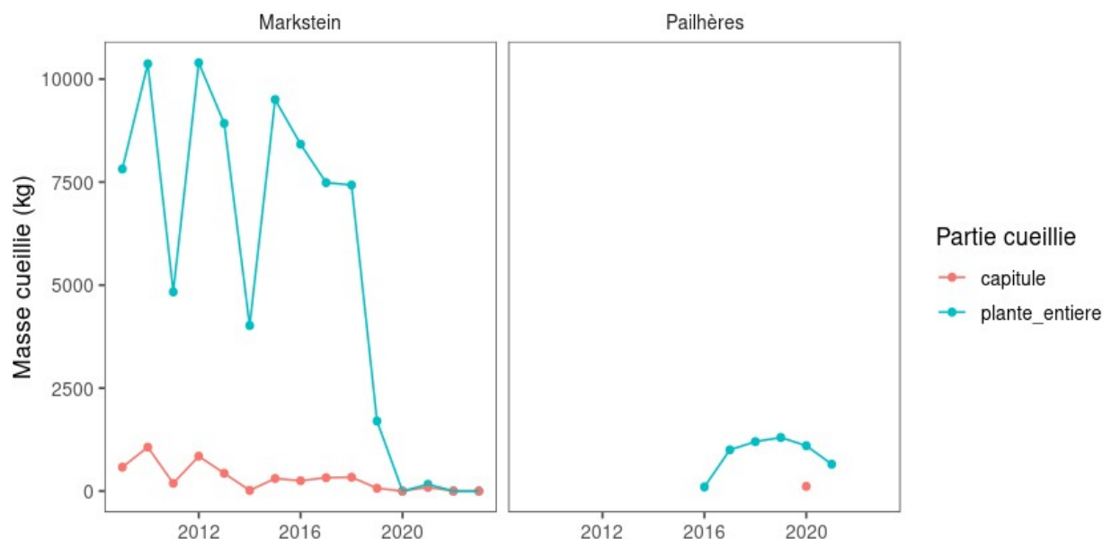
Figure 20 : Suivi de la masse d'arnica frais cueilli (capitule et plante entière). À gauche sur le site du Markstein depuis 2009. À droite, sur le site de Pailhères entre 2016 (année de test) et 2021. Des cueillettes non autorisées par d'autres équipes de cueilleurs ont cependant eu lieu et ne sont pas présentées ici. D'après des données de Garreta et al. (2022).
