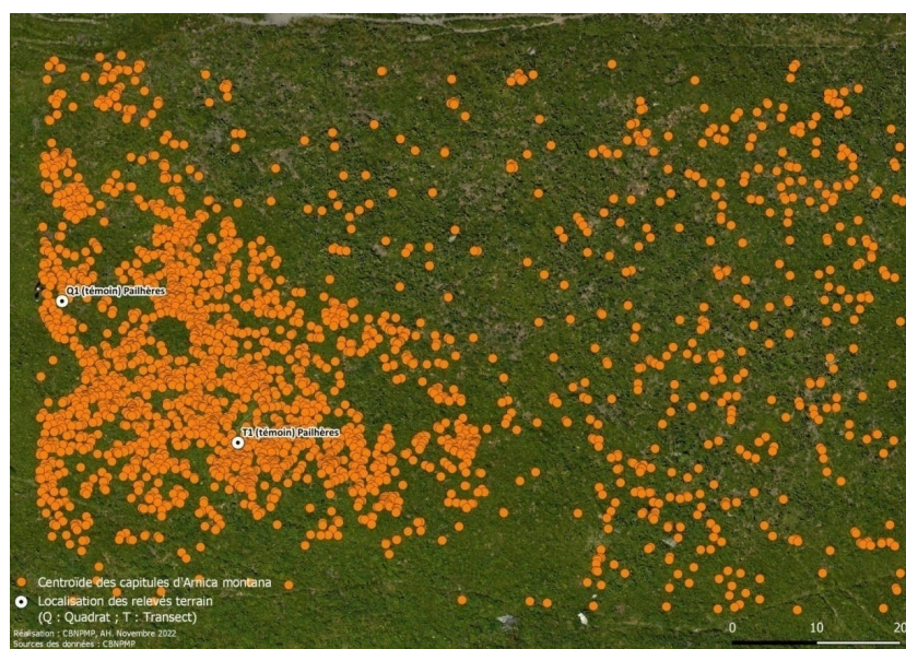
Figure 19 : Cartographie de la répartition de l'arnica en 2022 sur une partie du site de cueillette de Pailhères, à partir de l'imagerie drone. L'hétérogénéité spatiale de la ressource est clairement visible. Tiré de Hamdi (2022)
