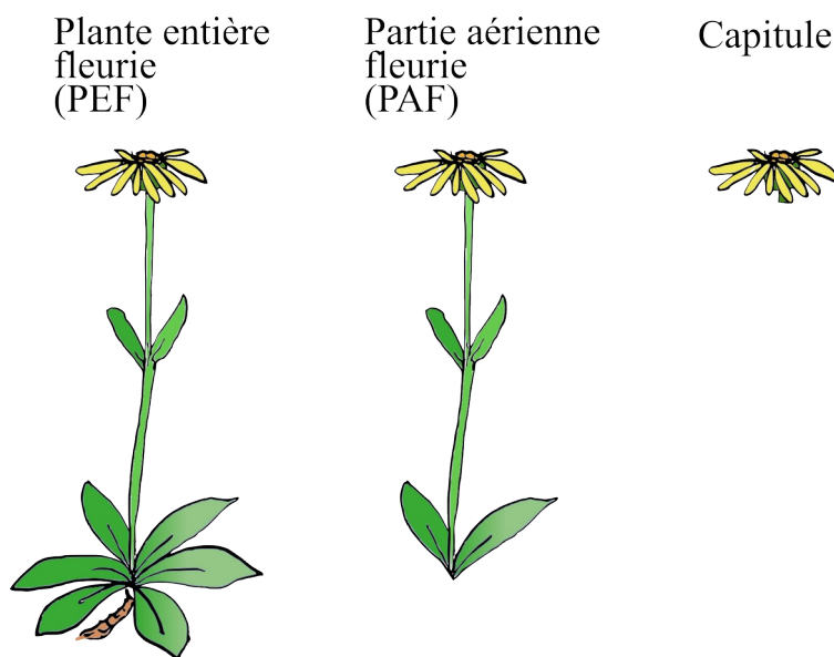
Figure 8 : Les différentes modalités de cueillette de l'arnica
