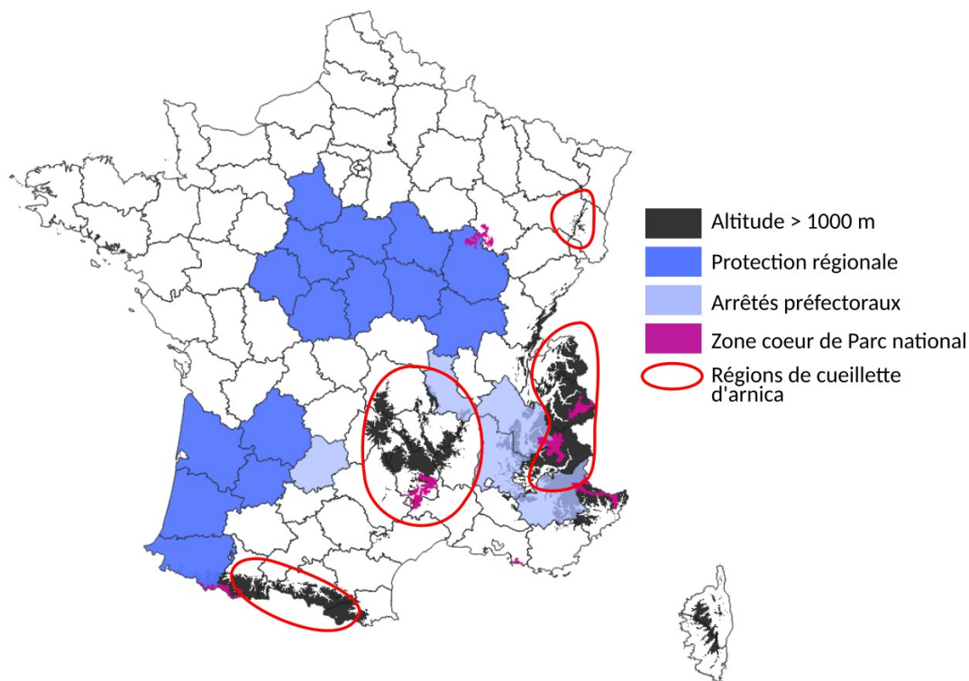
Figure 7 : Les principales régions de cueillette d'arnica en France, délimitées par des cercles rouges.
